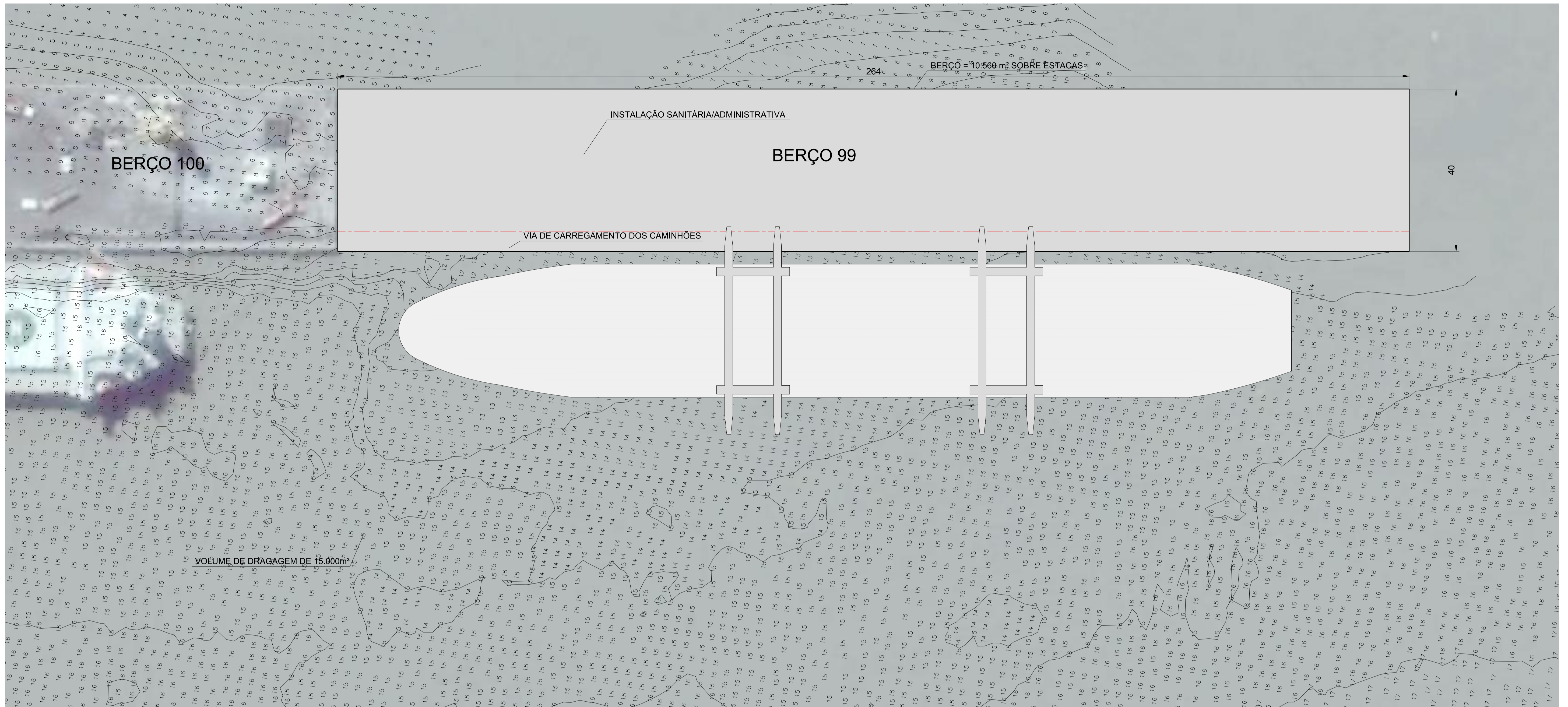
BERÇO 99 - BATIMETRIA ESCALA: 1:500
